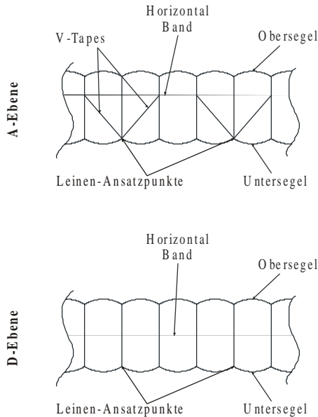
Abbildung 1: Honeycomb-V-Tape System des UP Trango
