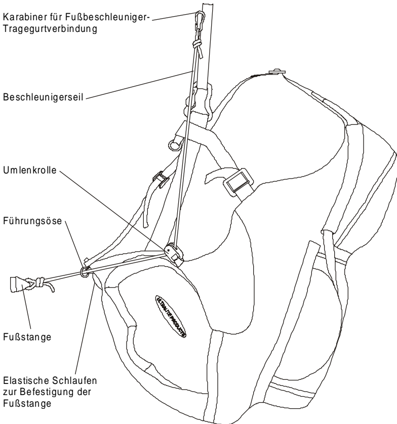
Abbildung 7: Beschleunigungssystem
