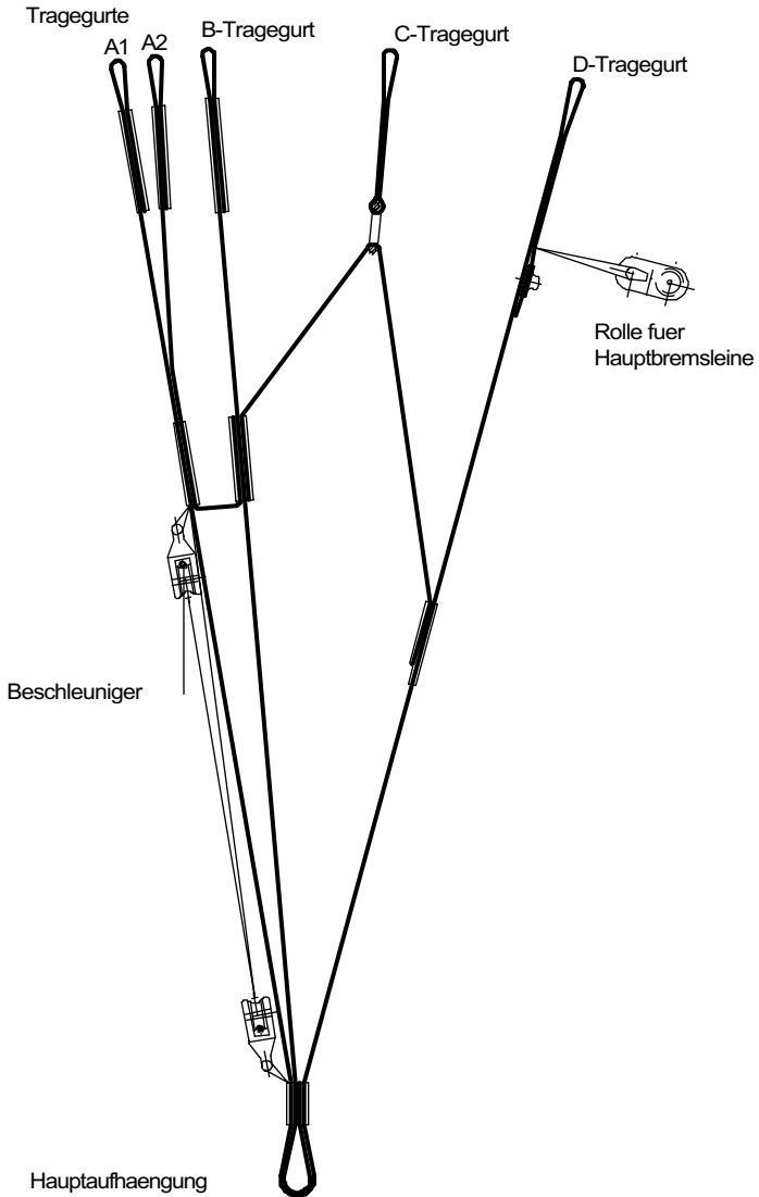
Abbildung 2: Tragegurt UP Makalu 2
