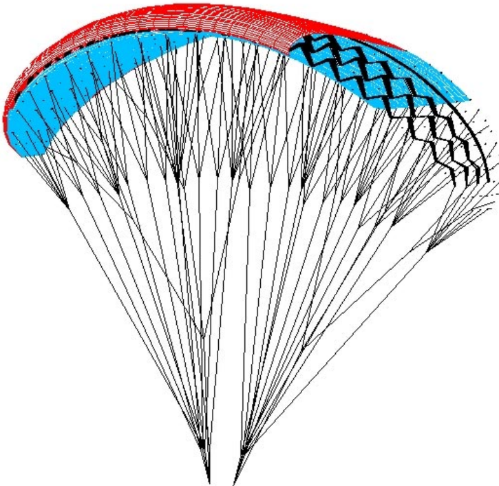
Abbildung 1: Segelaufbau des UP Makalu 2 mit Rippen und V-Tapes
