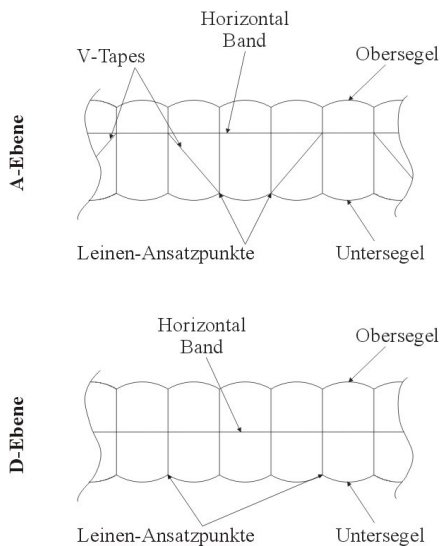
Abbildung 1: Honeycomb-V-Tape System des UP Kantega
