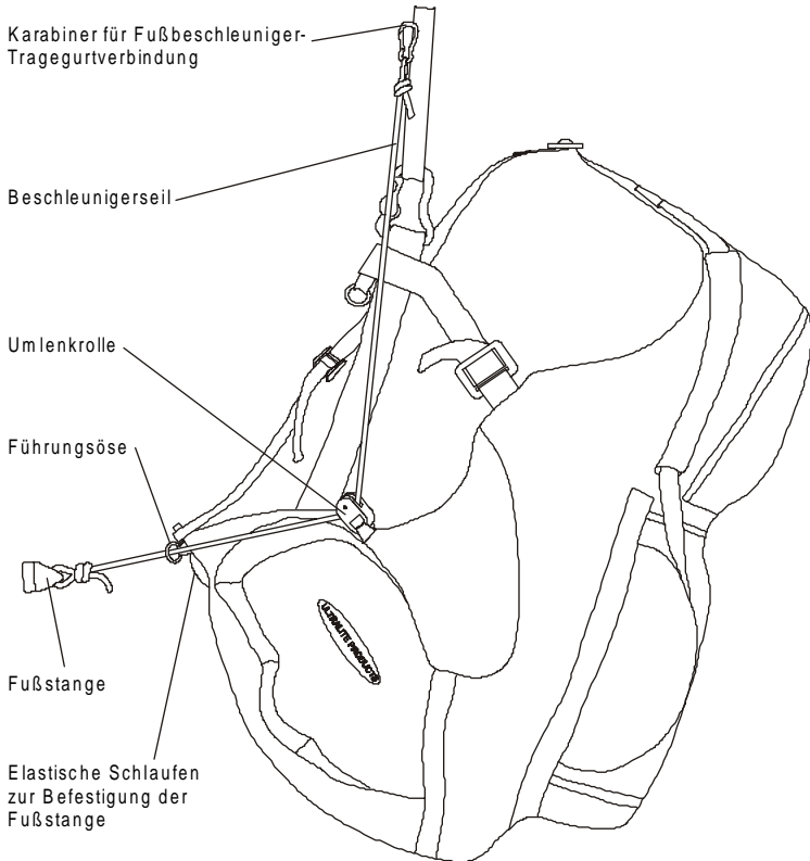
Abbildung 7: Beschleunigungssystem
