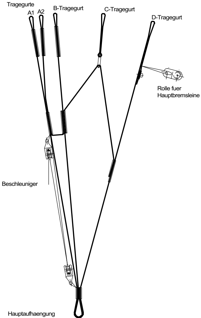
Abbildung 2: Tragegurt UP Kantega
