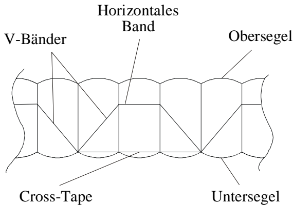
Abbildung 1: Segelaufbau
