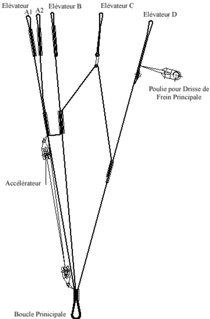
Illustration 2 : Elévateurs UP Makalu
