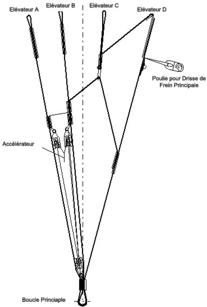
Illustration 2 : Elévateurs UP Summit 2
