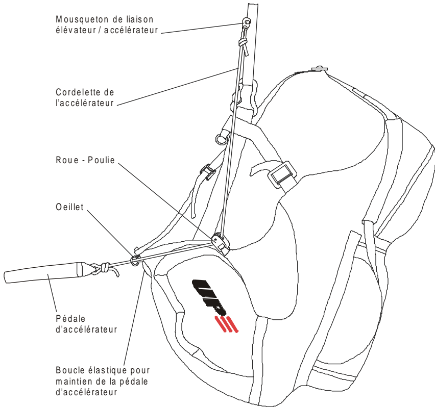
Illustration 7: Composants de l'accélérateur et passage de la cordelette
