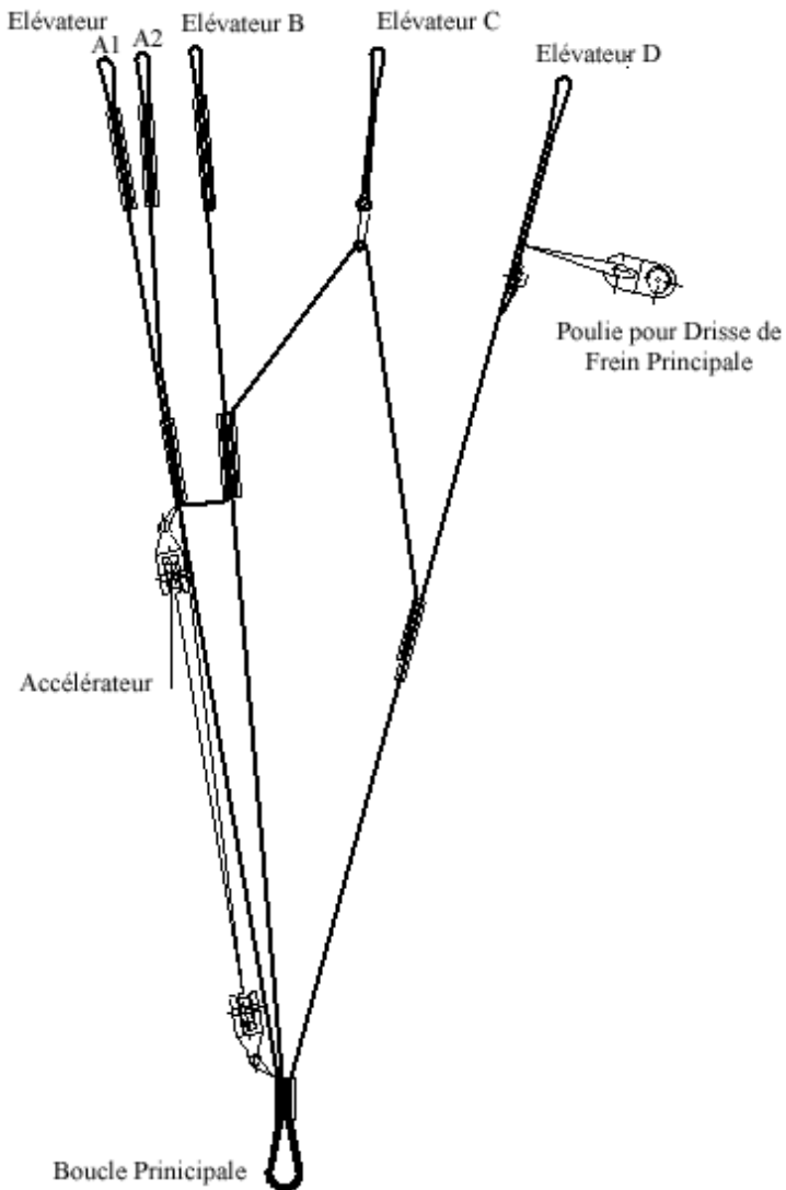
Illustration 2 : Elévateurs UP Makalu 2
