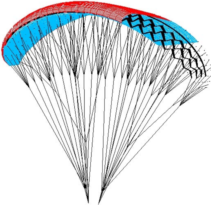
Illustration 1 : Construction de la voile, avec renforts et cloisons en V.
